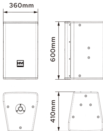
DS812外形尺寸图
