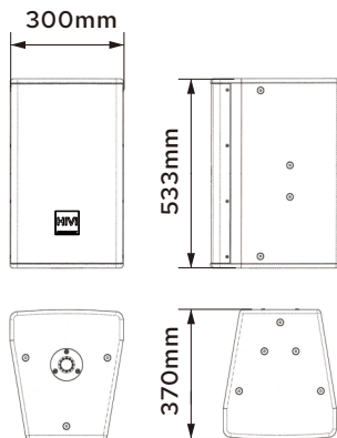
DS810外形尺寸图
